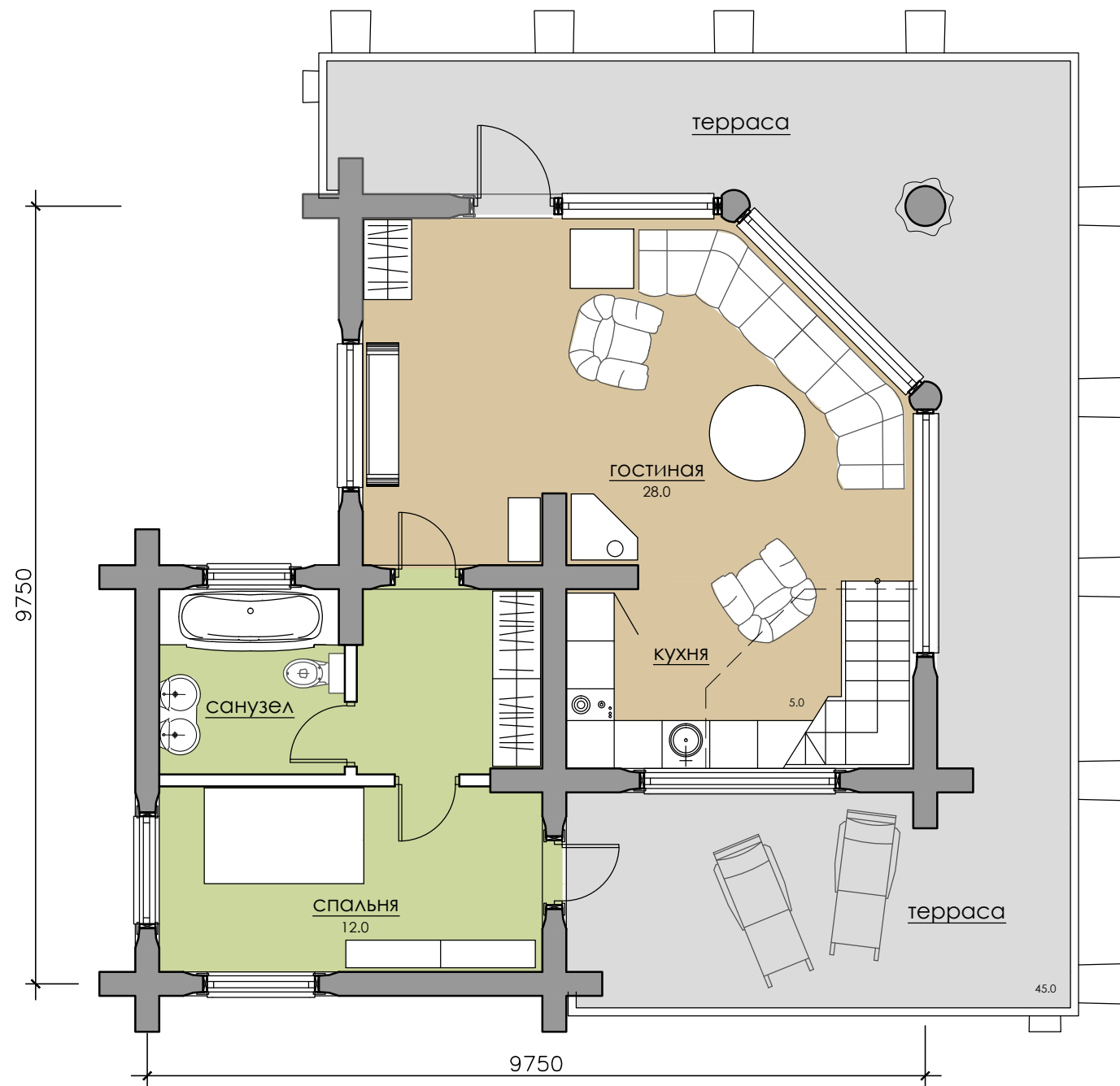
план 1 этажа 58.0 (+45.0)
